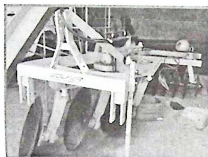
Implementos que acompanham o trator: arado hidráulico reversivo e grade hidráulica niveladora
